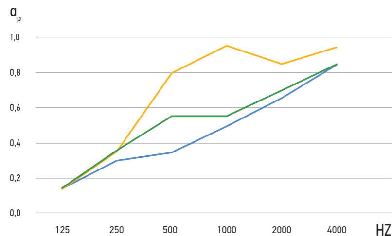
Elnyelés értékelése | Evaluation of absorption
