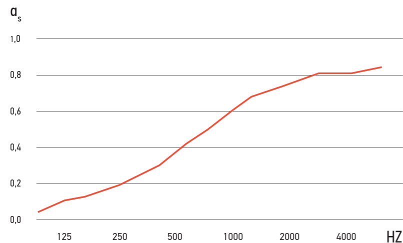
Az akusztikus hab hangelnyelő képességének mérése | Measurement of the sound absorption of acoustic foam
